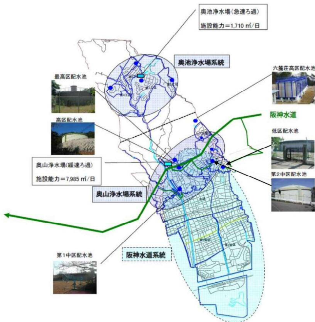
図 2.4 水道施設の概要
