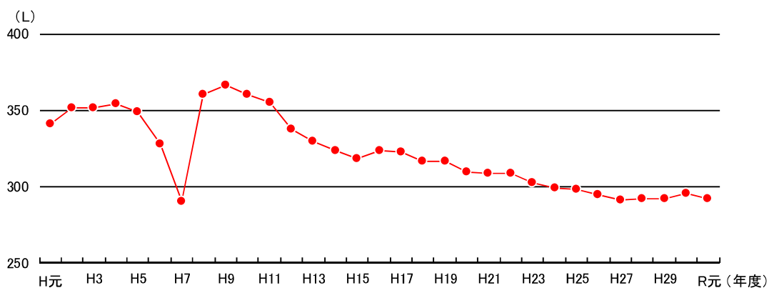
図 2.10 一人一日平均有収水量の推移
