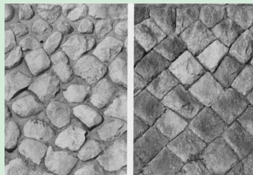
芦屋川の護岸左：野面積み 右：谷積み
