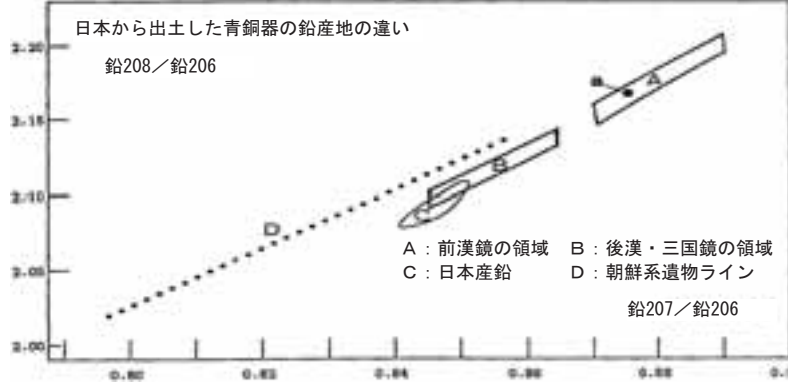
日本出土青銅器の鉛同位体比分布図 【馬淵2007『考古学と自然科学』55号から】
