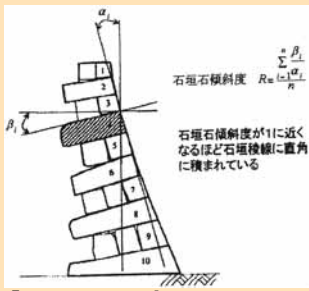
『玉野のほかに2009』から 石垣石控比・石垣石加工度・石垣傾斜度
