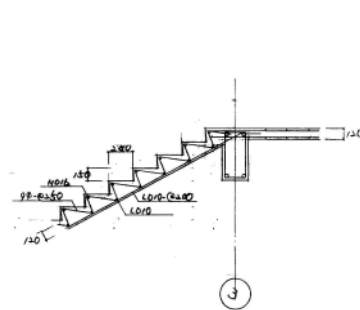
A. 階段詳細図 1/30
