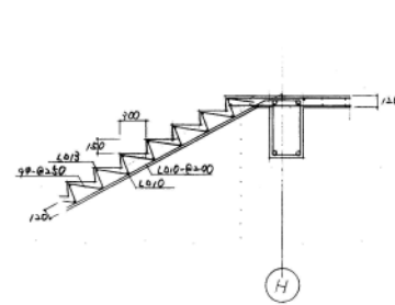
B. 階段詳細図 1/30
