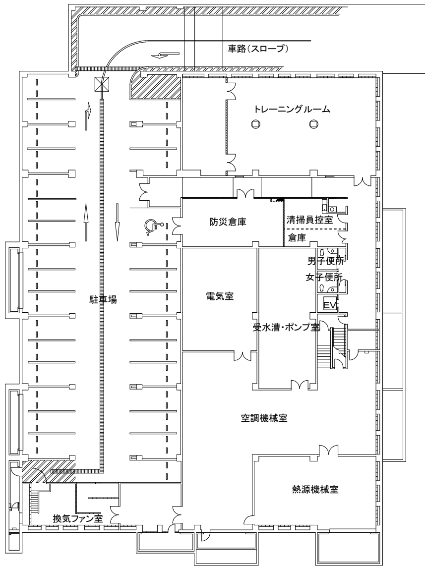
地階平面図(改修後)
