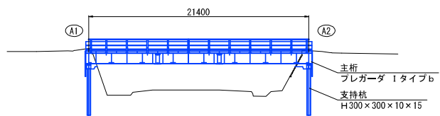
仮橋横断面図 S=1:500
