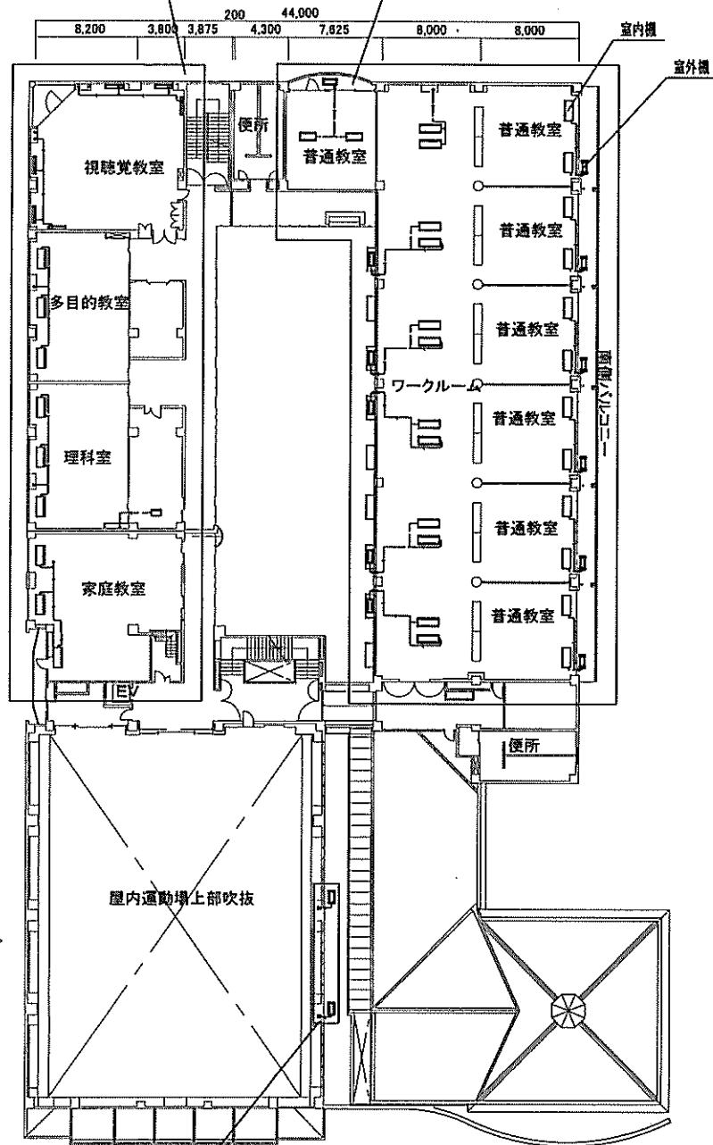
空調設備 3階平面図 (改修後)
