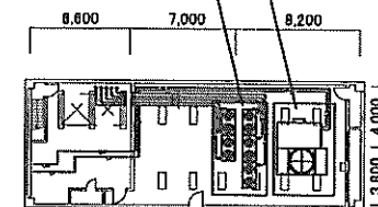
空調設備 塔屋階平面図 (改修後)
