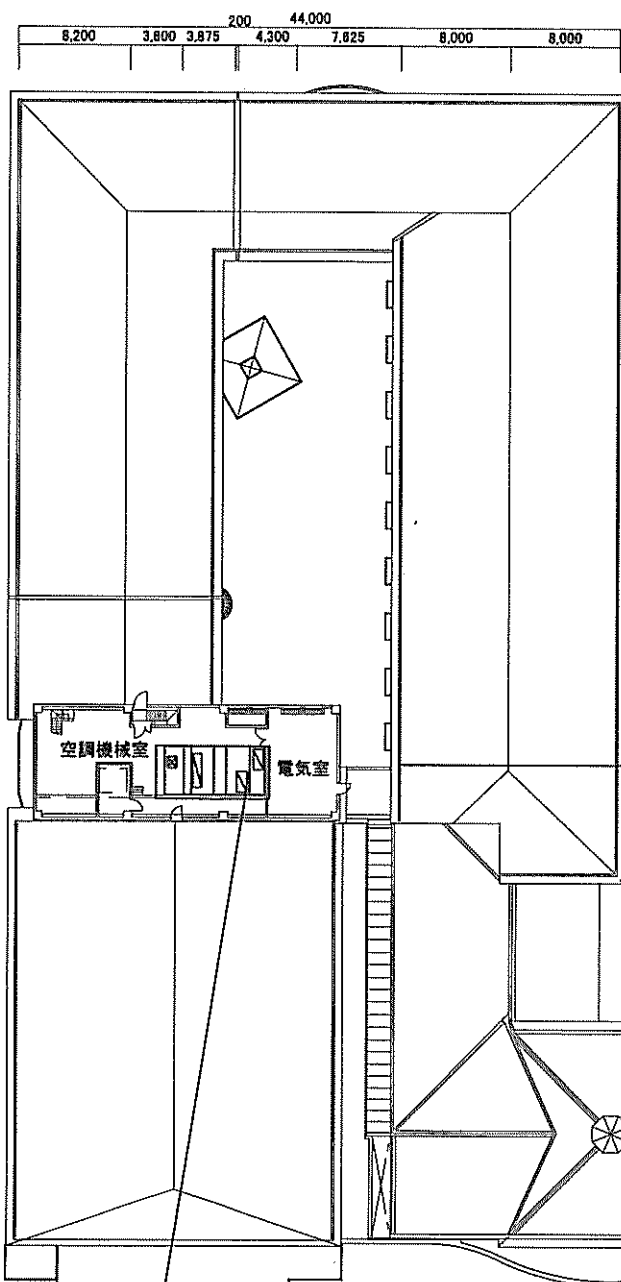
空調設備 塔屋階平面図 (改修後)
