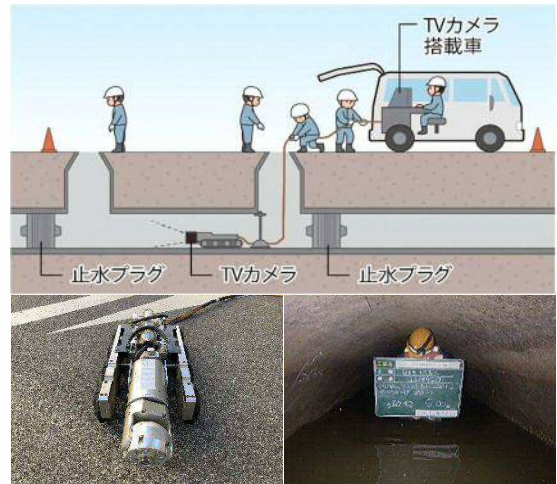
写真5 管路の調査
