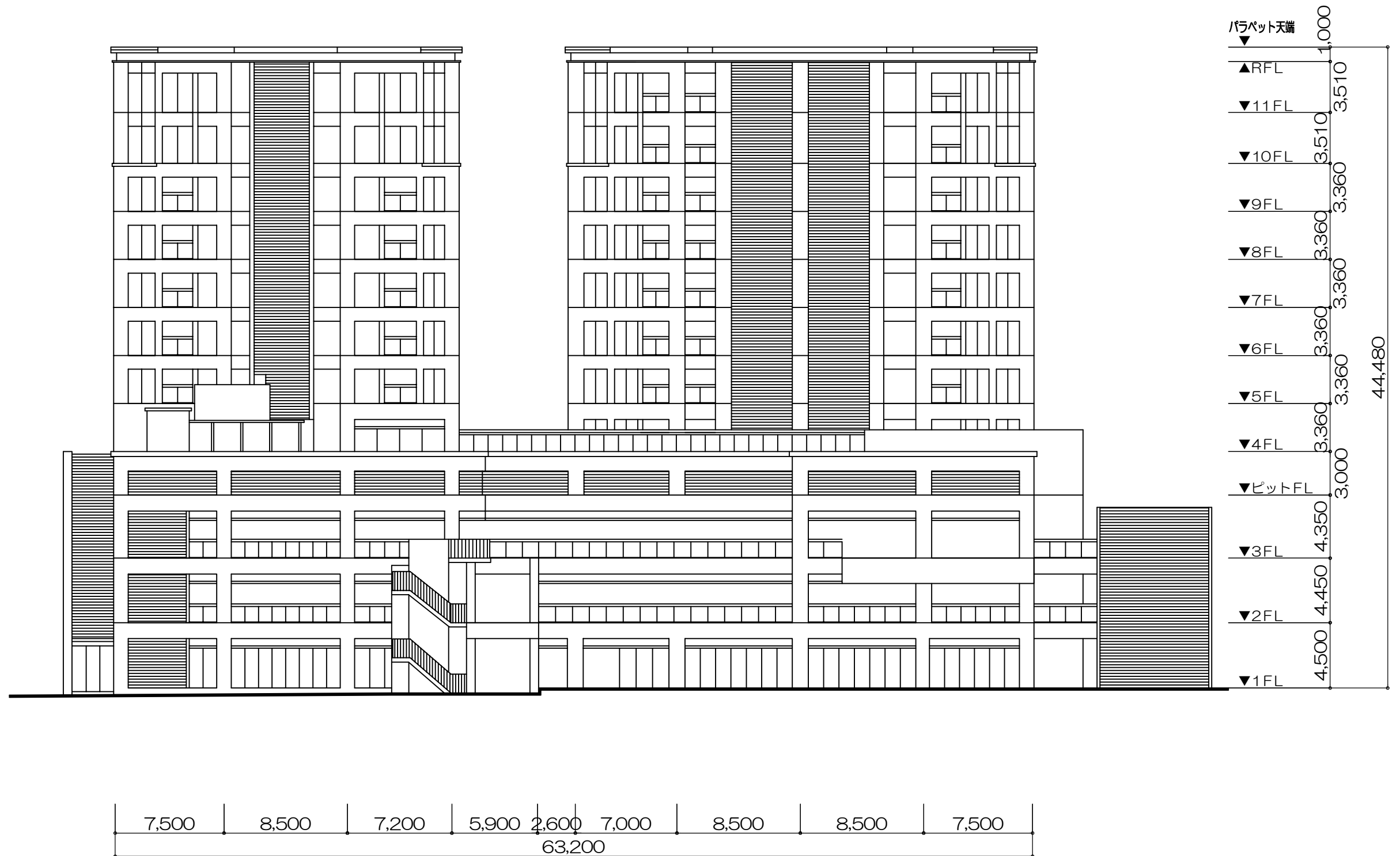
JR芦屋駅南地区第二種市街地再開発事業 北立面図 1/300
