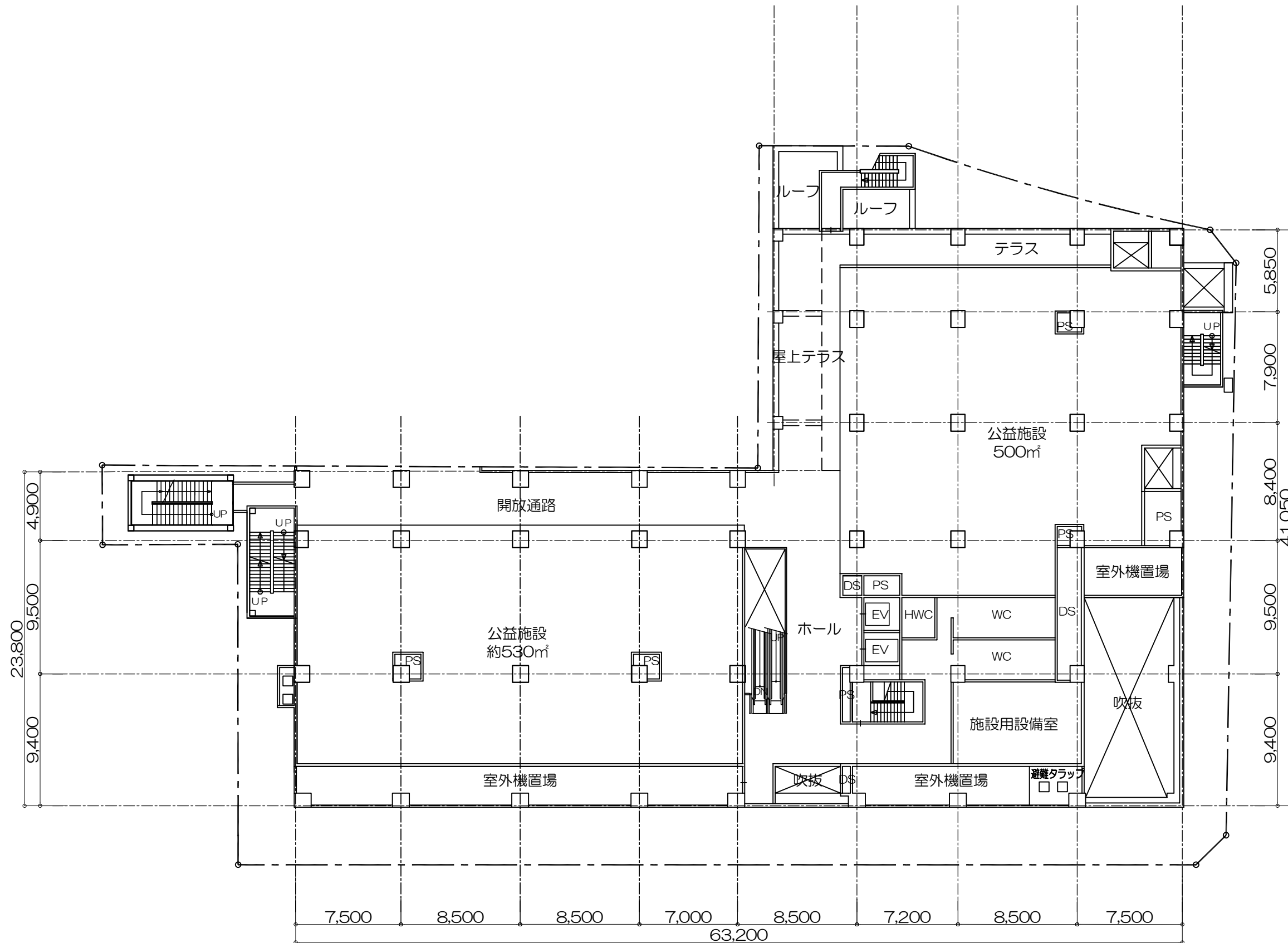
JR芦屋駅南地区第二種市街地再開発事業 3階平面図 1/300
