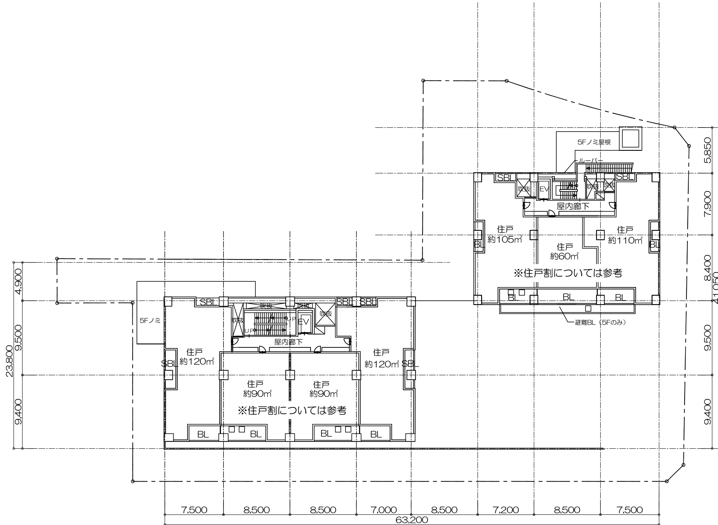
JR芦屋駅南地区第二種市街地再開発事業 5~11階平面図 1/300
