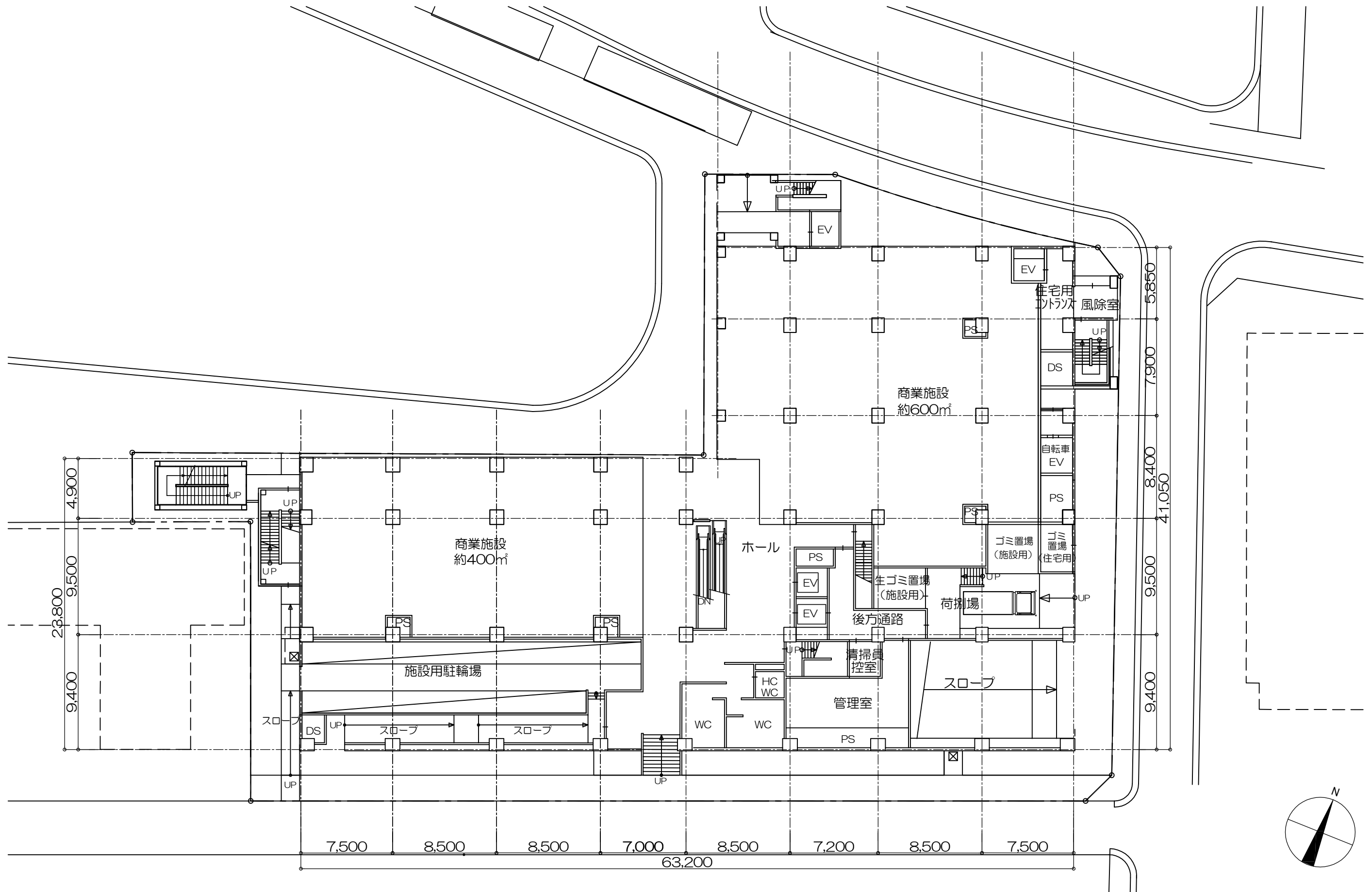
JR芦屋駅南地区第二種市街地再開発事業 1階平面図 1/300
