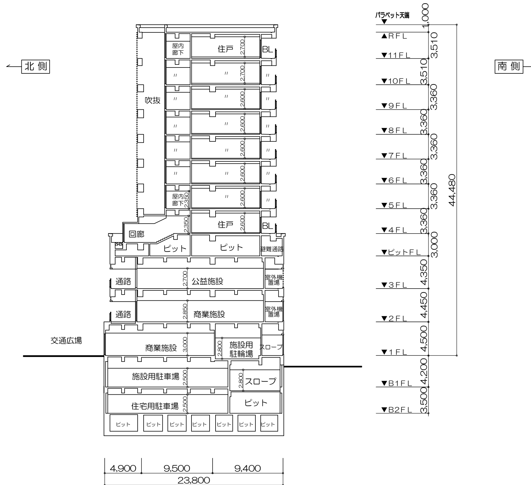
JR芦屋駅南地区第二種市街地再開発事業 南-北断面図 1/300
