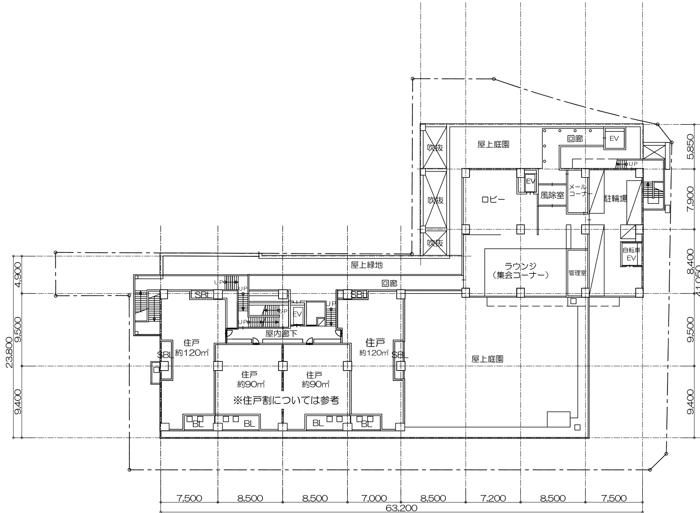
JR芦屋駅南地区第二種市街地再開発事業 4階平面図 1/300
