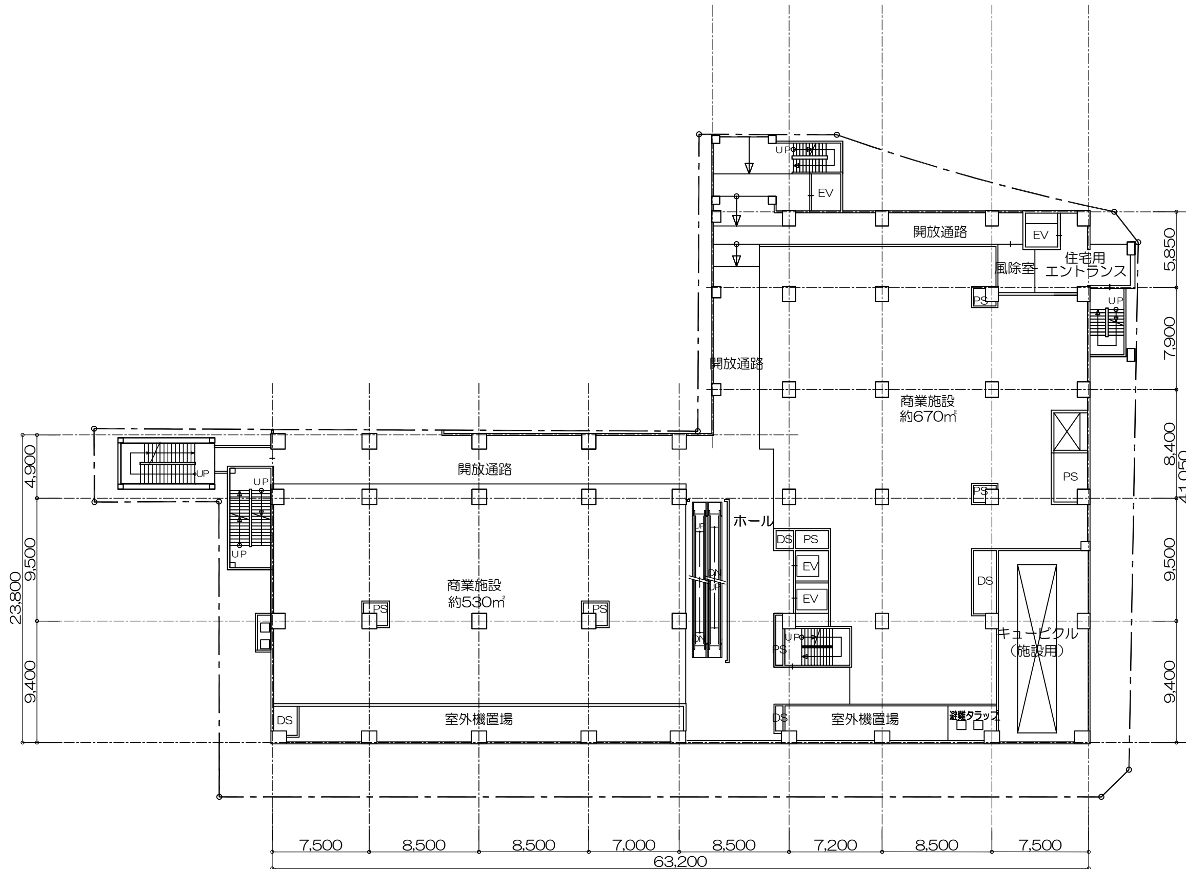
JR芦屋駅南地区第二種市街地再開発事業 2階平面図 1/300
