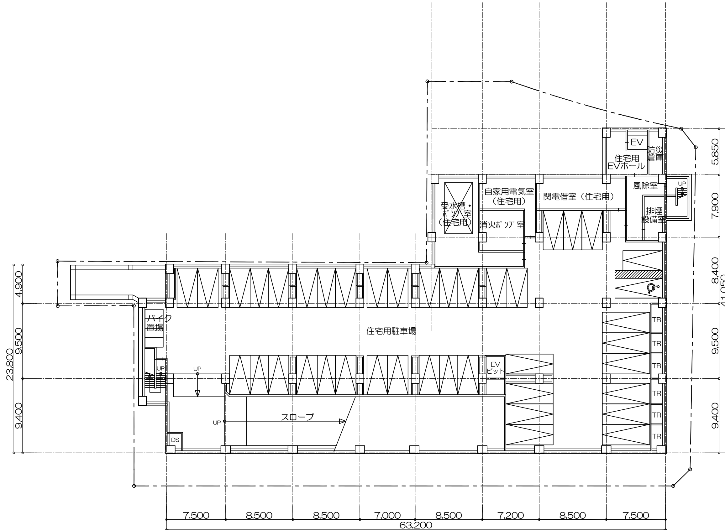
JR芦屋駅南地区第二種市街地再開発事業 B2階平面図 1/300
