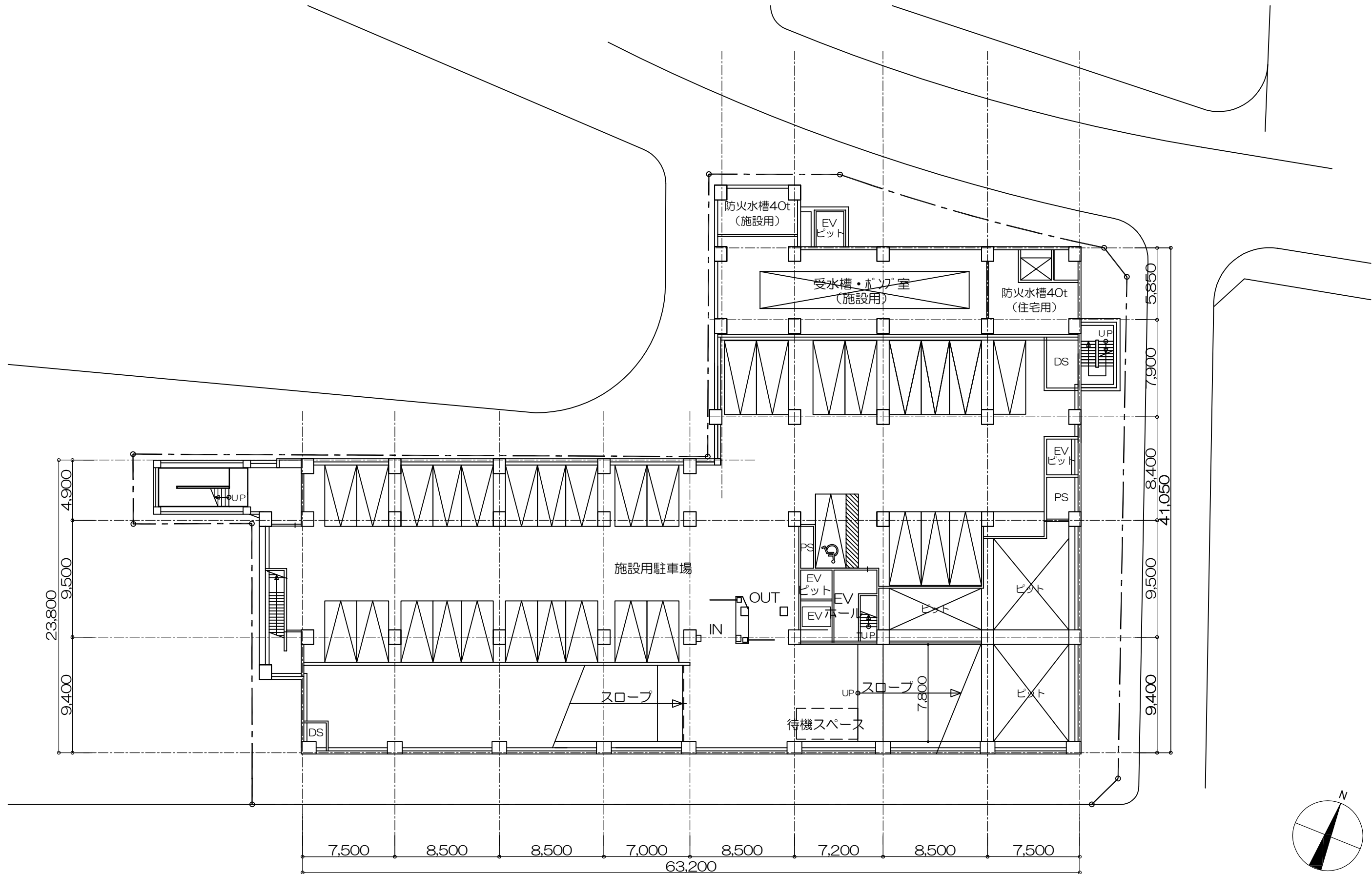
JR芦屋駅南地区第二種市街地再開発事業 B1階平面図 1/300
