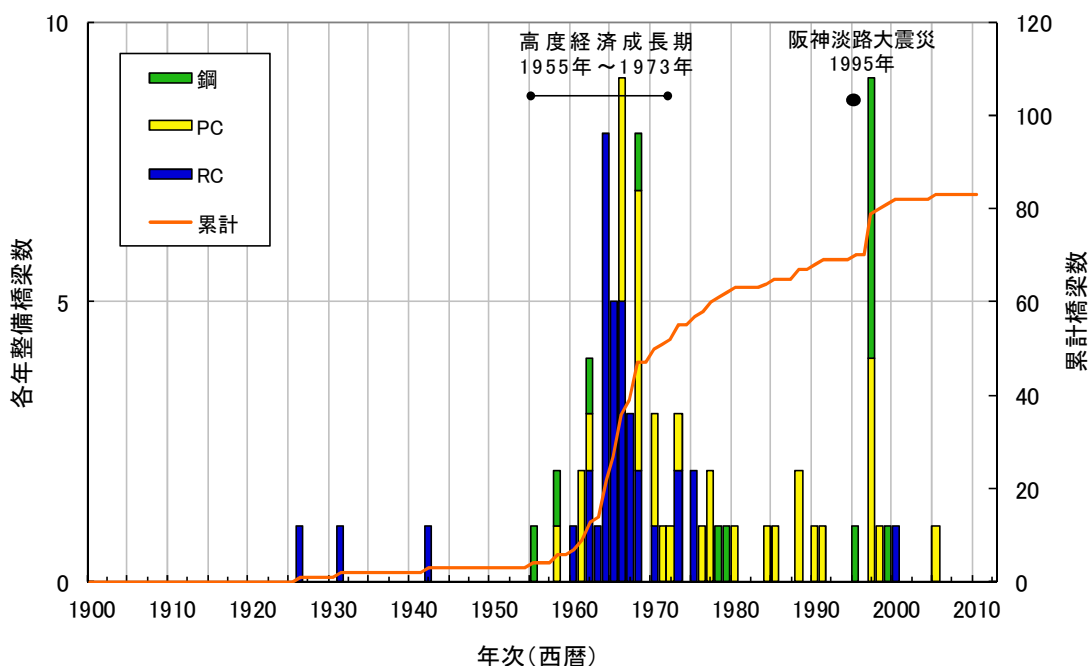
高齢化道路橋の分布の変化
